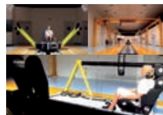
衝突試験機
